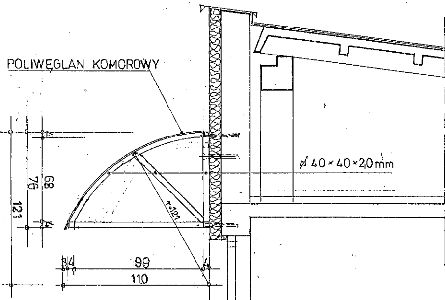
przekrój a-a
