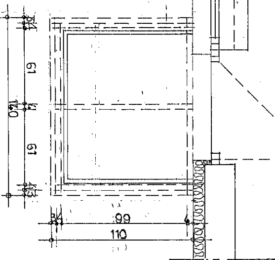
widok czołowy 1:20
